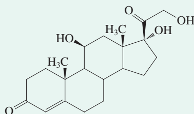
Cortisol
