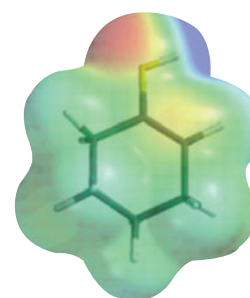
Enol
