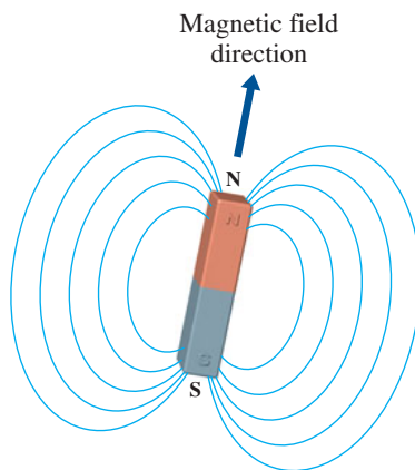
Bar magnet
