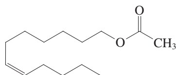
(Z)-7-Dodecenyl acetate
