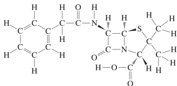
Benzylpenicillin
