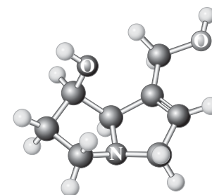
Retronecine
