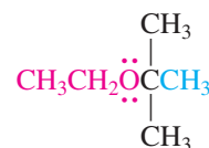
2-Ethoxy-2-methylpropane
