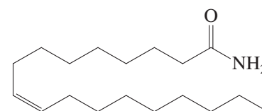
(Z)-9-Octadecenamide
