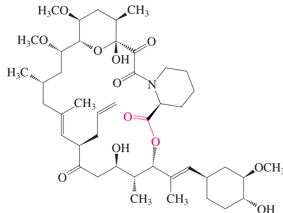
Tacrolimus (FK-506)
