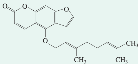
Bergamottin
