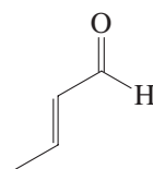
( E )-2-Butenal
