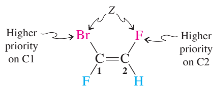
(Z)-1-Bromo-1,2-difluoroethene
