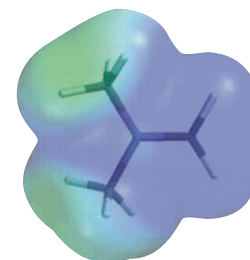
Iminium ion
