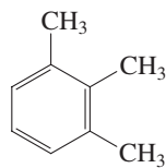
1,2,3-Trimethylbenzene
