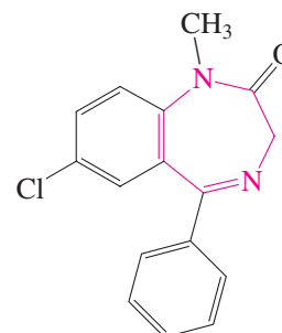
Diazepam (Valium)
