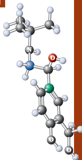
S-(+)-Albuterol
