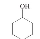
Cyclohexanol
