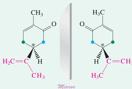
Carvone enantiomers
