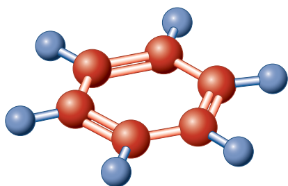
Benzene
