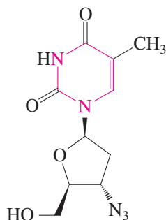
Zidovudine (AZT)
