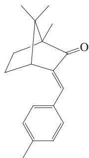
4-MBC
