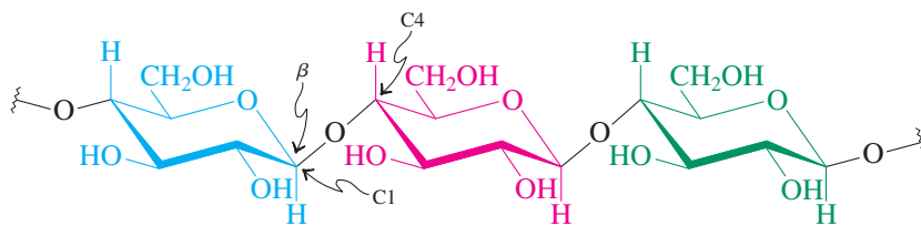
Cellulose
