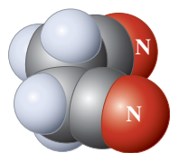
Butanedinitrile (Succinonitrile)
