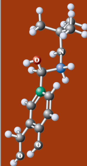
R-(-)-Albuterol
