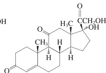
Cortisone
