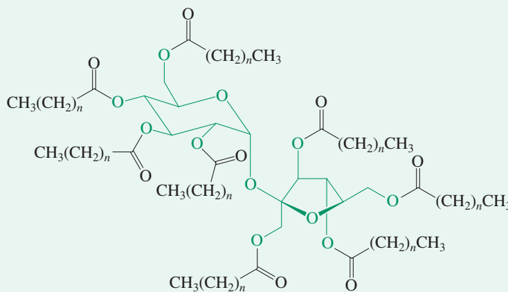
Olestra
