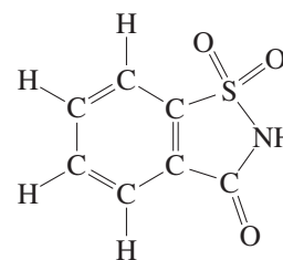
Saccharin
