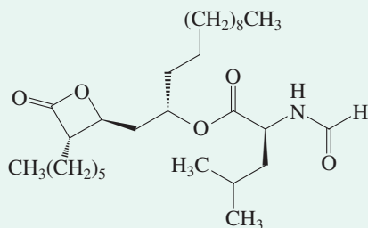
Orlistat (Xenical)
