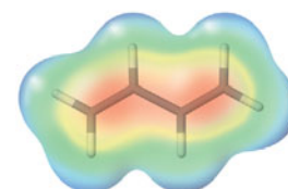
1,3-Butadiene (Conjugated)
