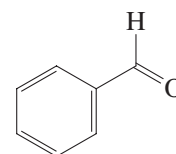
Benzenecarbaldehyde (Benzaldehyde)
