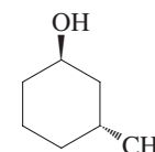
trans -3-Methylcyclohexanol
