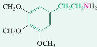
Mescaline (Hallucinogen)
