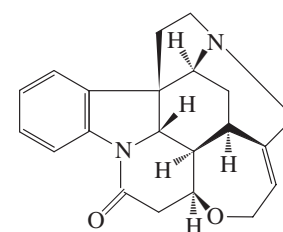
Strychnine
