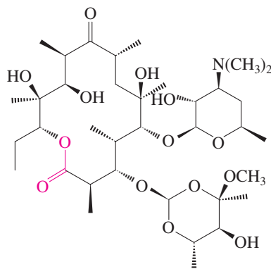
Erythromycin A
