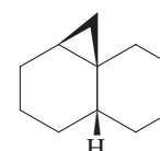
Tricyclo[5.4.0 1,3 .0 1,7 ]undecane
