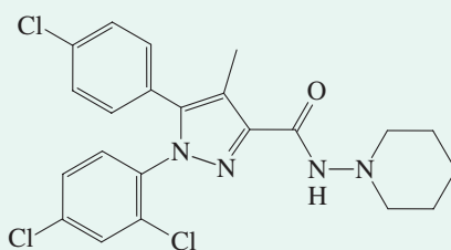
Rimonabant
