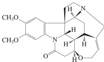
Brucine
