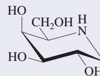
Migalastat
