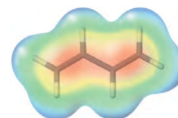
1,3-Butadiene (Conjugated)
