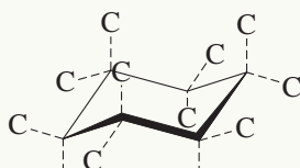
Diamond: sp^3
