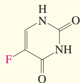
5-Fluorouracil (Fluracil)
