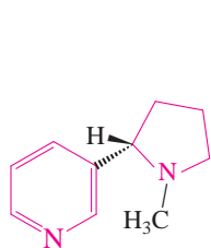
Nicotine
