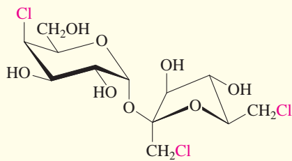
Sucralose
