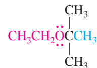
2-Ethoxy-2-methylpropane
