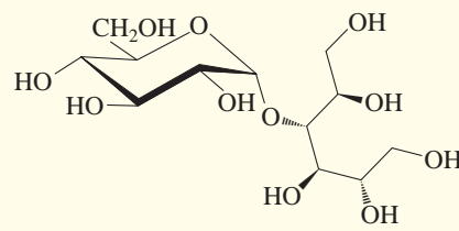
Maltitol (Glucopyranosylglucitol)
