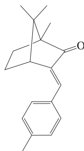
4-MBC
