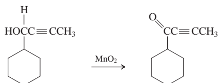
1-Cyclohexyl-2-butyne-1-one
