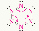
Hexaazabenzene (Hexazine)
