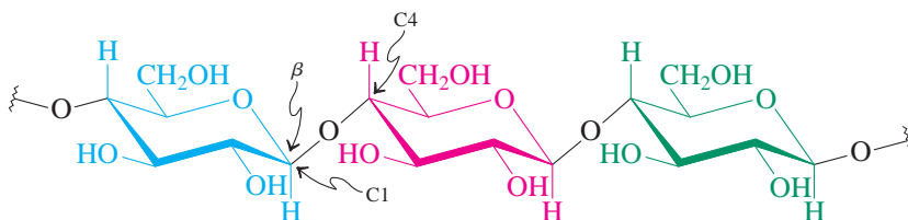
Cellulose
