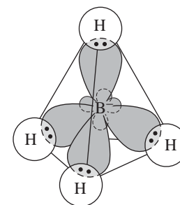
Borohydride ion
