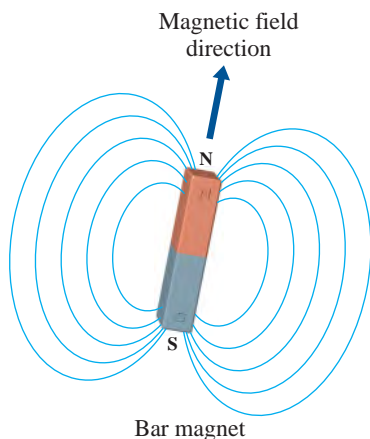
Bar magnet
