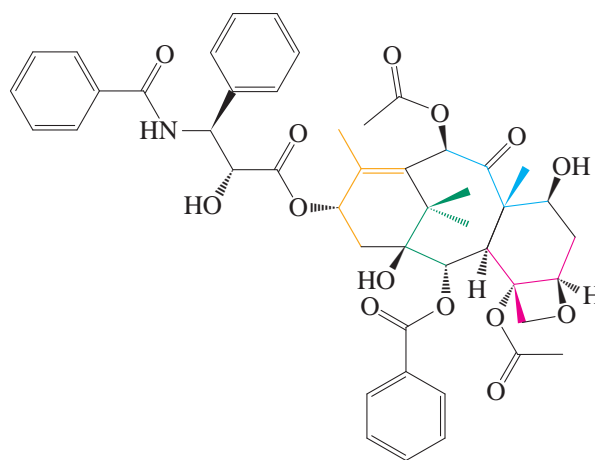
Taxol
