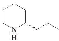
(+)-Coniine
