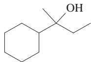
2-Cyclohexyl-2-butanol
